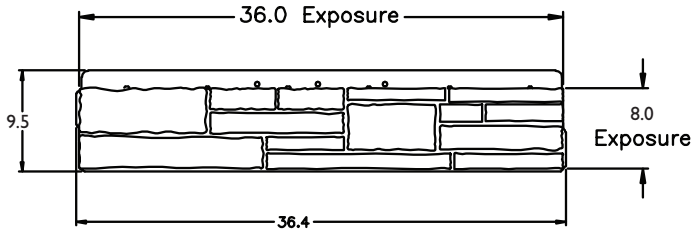
FIGURA 6 - TOPE DE RECUBRIMIENTO
