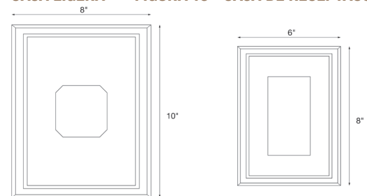
FIGURA 15 - CAJA LIGERA FIGURA 16 - CAJA DE RECEPTÁCULOS
