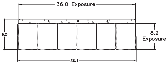
FIGURA 8 - PANEL DE MOLDURA
